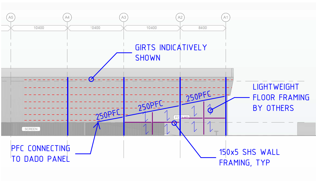
ELEVATION 1
