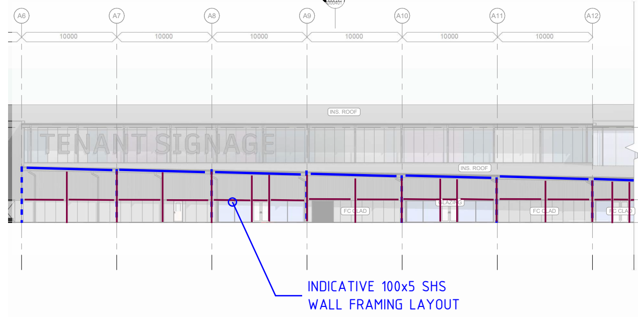
ELEVATION 2
